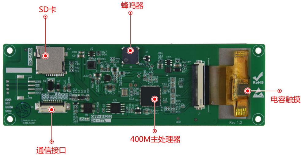
图 1-3 硬件配置图
