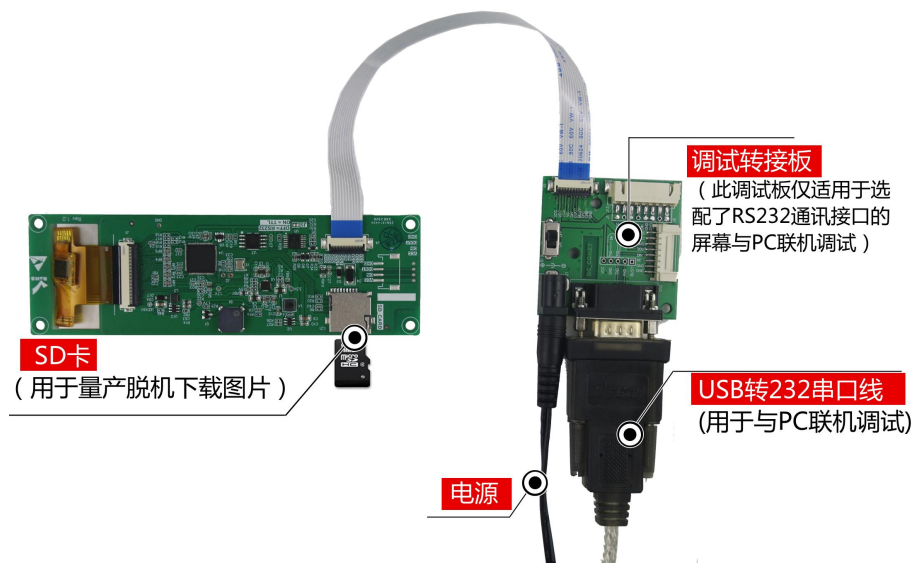
图 1-4 调试工具图
