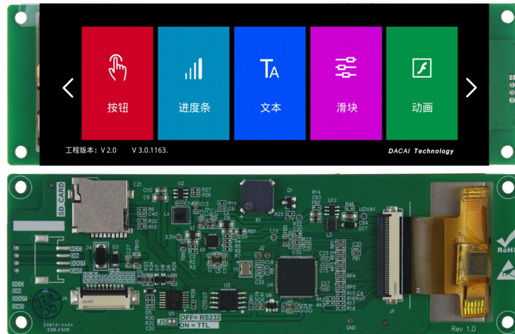
图 1-1 4.6 寸电容触摸参考图
